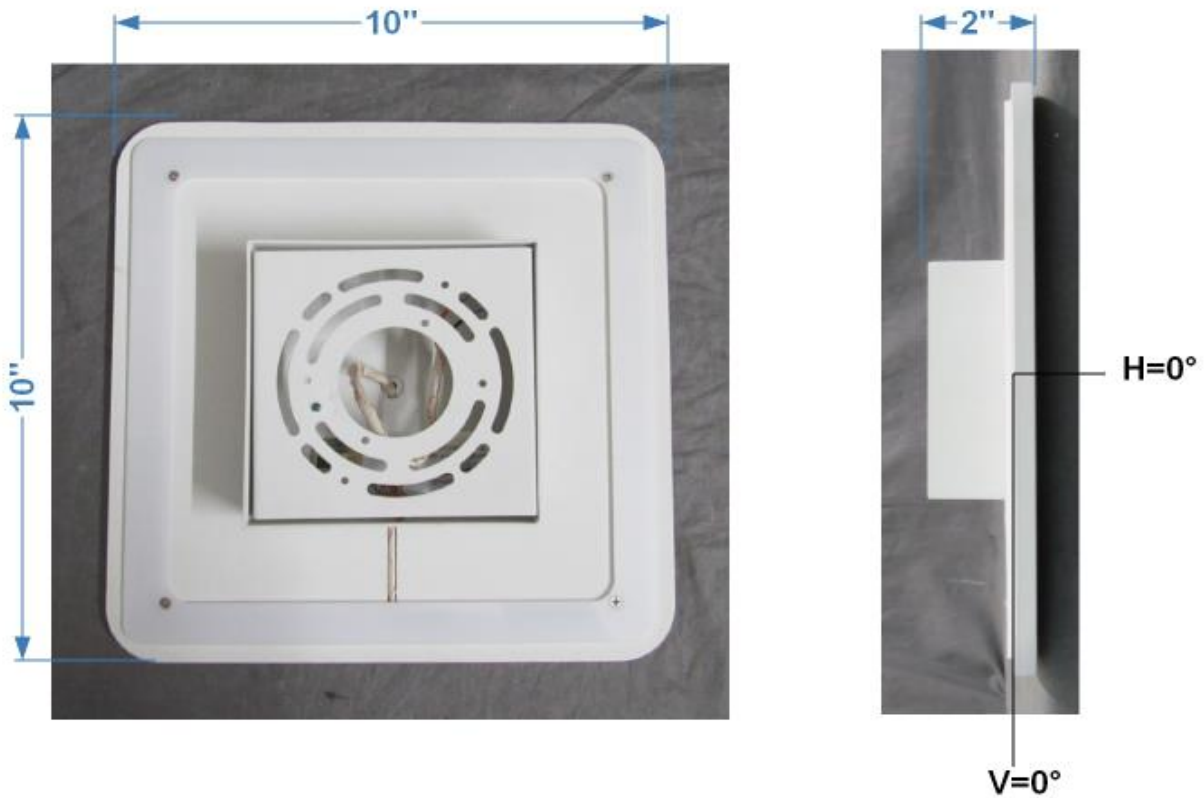
FIG. 1 LUMINAIRE
