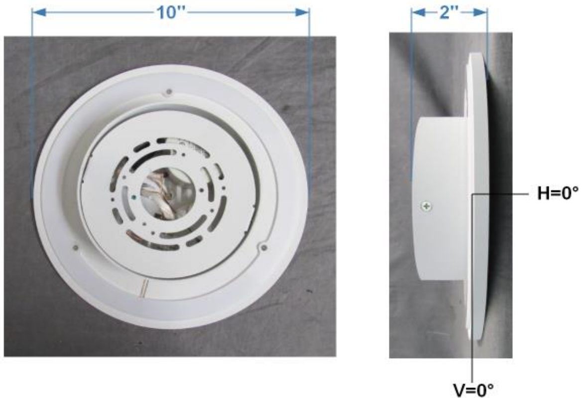
FIG. 1 LUMINAIRE
