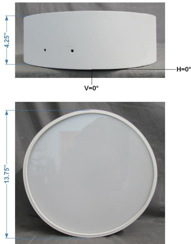
FIG. 1 LUMINAIRE
