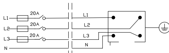
3 phase 120V 3x20A Max
