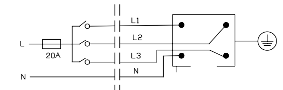
1 phase 120V 20A Max
